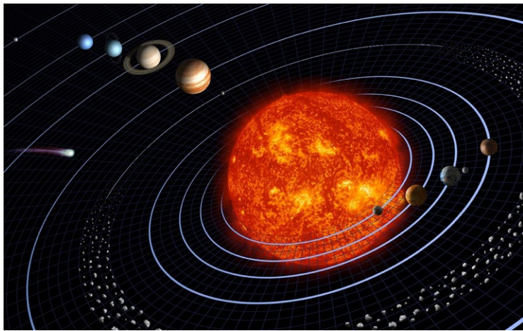
太陽系。
