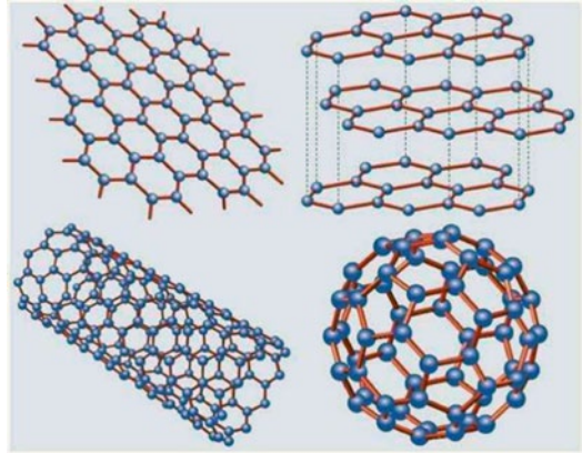
四種碳材料：石墨烯、石墨、碳奈米管（左下）與富勒烯（右下）。
