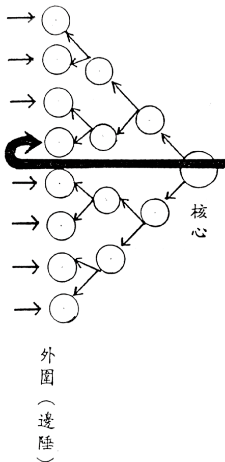
圖2：核融合(聚變)形勢示意簡圖。
