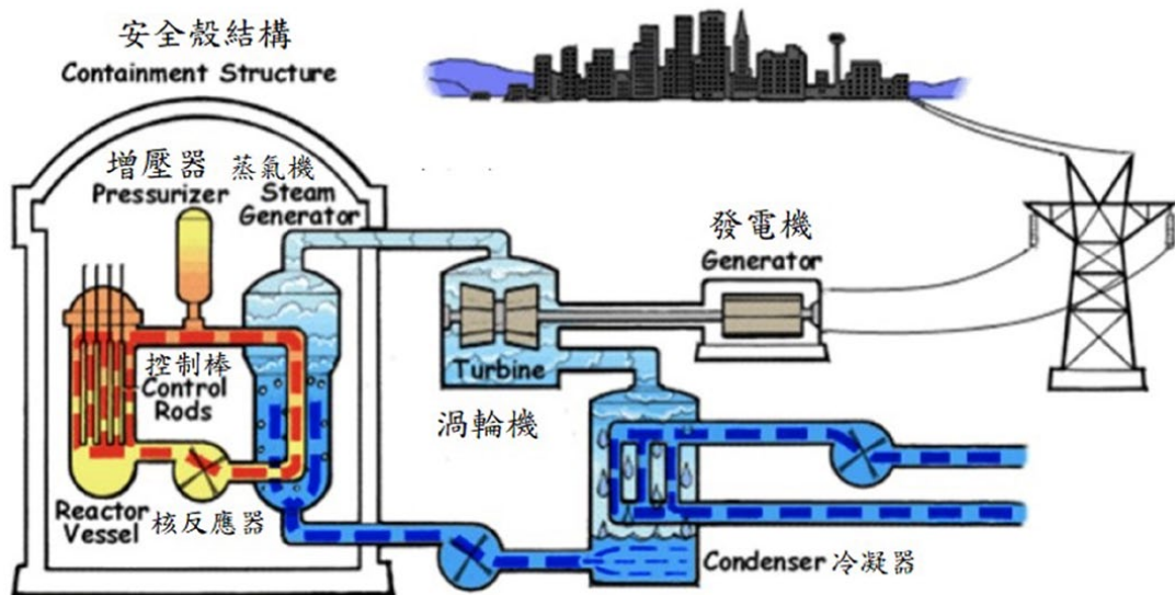
核電廠結構。
