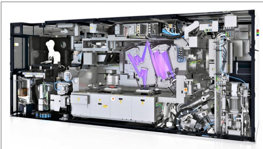
光刻機的原理其實像幻燈機一樣簡單，就是把光透過帶電路圖的掩膜（Mask，也叫光罩）投影到塗有光敏膠的晶圓上。（取材自荷蘭ASML艾斯摩爾公司型錄）
