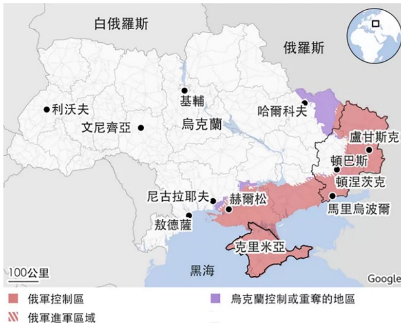
紅色區域（除克里米亞外）是俄羅斯目前佔領的烏克蘭領土，也是「公投入俄」的四州；紫色部分為烏克蘭 9 月反攻收復的領土。（圖片來源：戰爭研究所 Institute for the Study of War）
