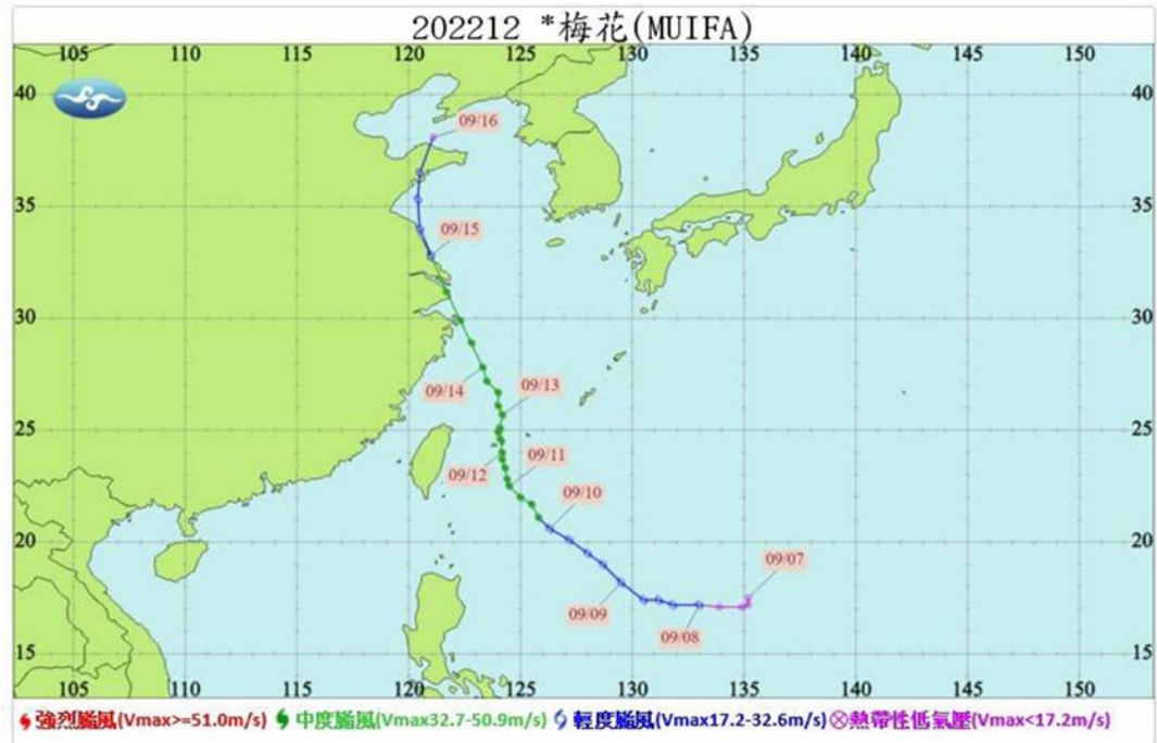
梅花颱風路徑圖。(梅花避開臺灣就增強為強颱，中心登陸四次，糾纏大陸8天，重創大陸沿海)
