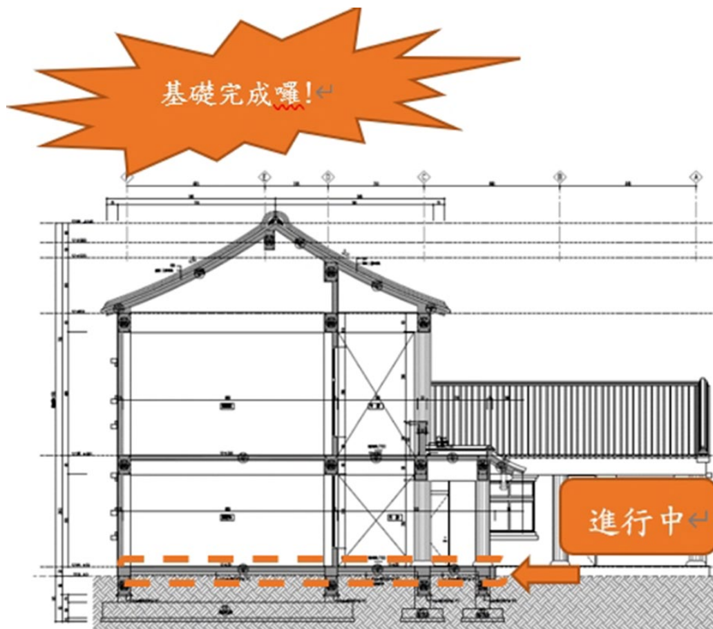
清涼內苑工程進度-說明：地上1樓樓版下防潮布及大底(PC)施工。
