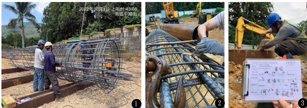
圖1/基樁鋼筋籠綁紮。
