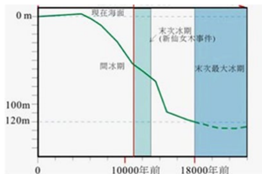
▲最後一次冰河時期，約2萬年前海平面下降圖。
