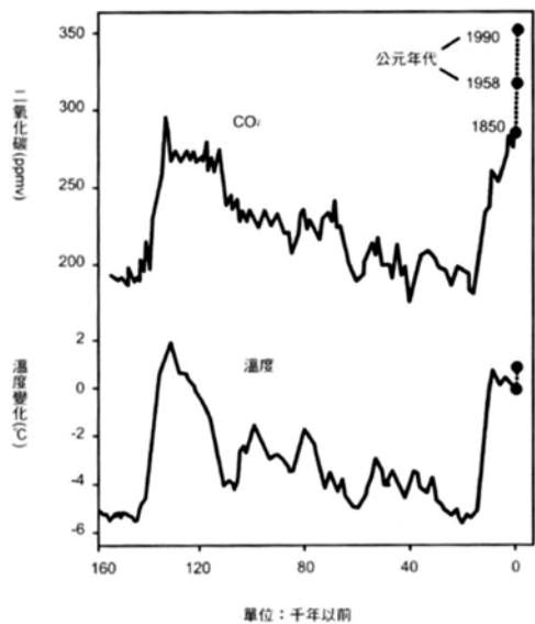
▲地球二氧化碳濃度與平均溫度升溫圖
