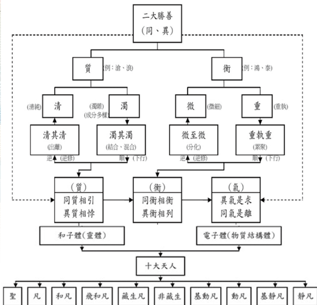
《天人親和真經》中的宇宙生命生化圖
